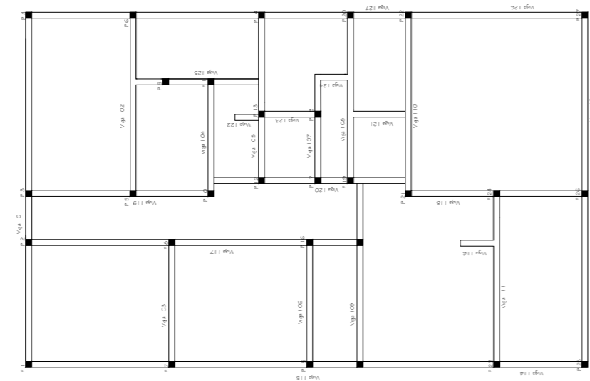
Planta de Localização dos Pilares e Cintas Escala 1/50
