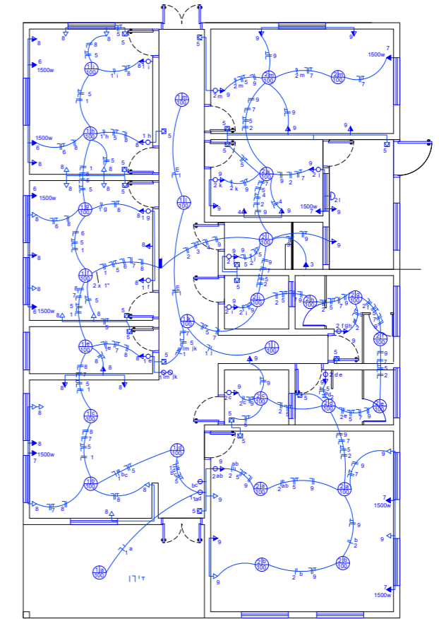
Planta das Instalações Elétricas Escala 1/50
