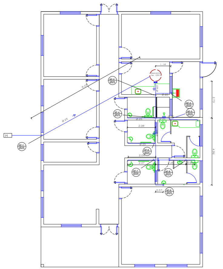
Planta das Instalações Hidrossanitárias - Água Escala 1/50
